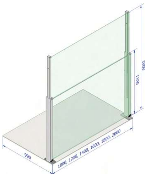
Wind Barrier ze stalową podstawą
