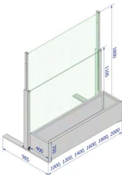
Wind Barrier z donicą aluminiową
