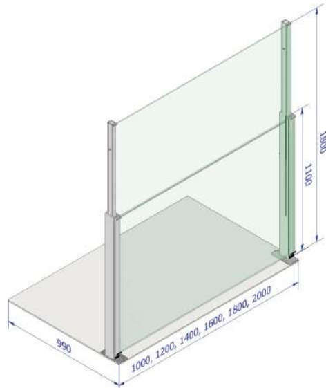
Wind Barrier mit Stahlständer
